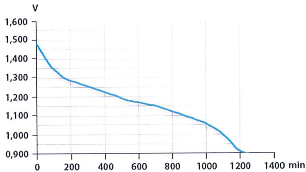
Portable lighting 4m/h 8h/d 3,9 ohm end 0,9V
