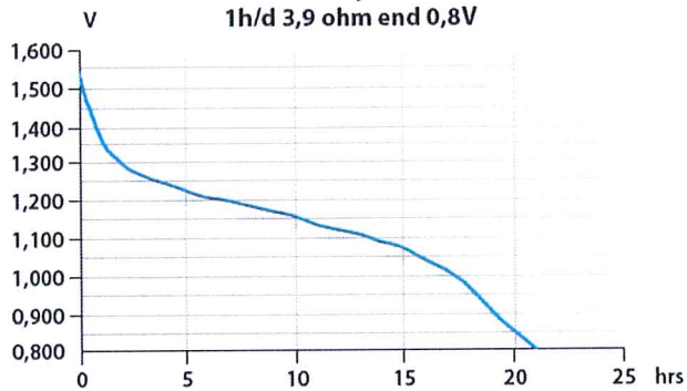
Toy 1h/d 3,9 ohm end 0,8V
